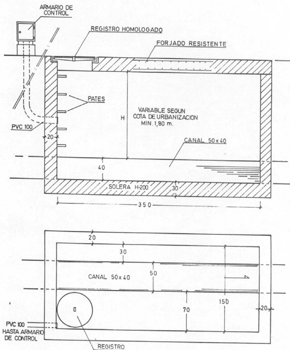
ARQUETA TIPO 2
