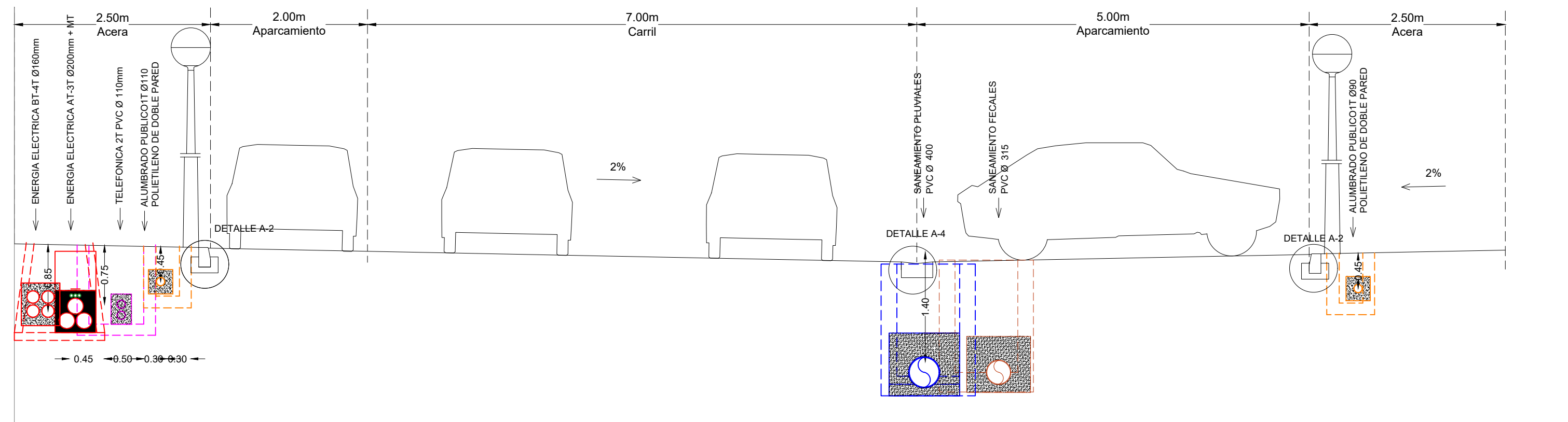
SECCION E-E
